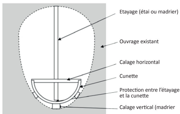
Figure 2 : Illustration d'une pose de cunette standards
